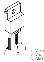
SE135N
